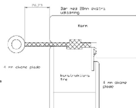
Fig. 3: Hængsler +20 med ekstra lang udladning giver plads op til 25 mm beklædning og op til 35 mm kombineret med fig.1
