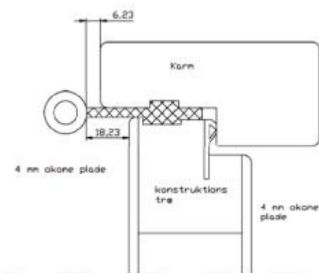
Fig. 1: Dørplade trukket tilbage fra karm giver plads til op til 15 mm beklædning
