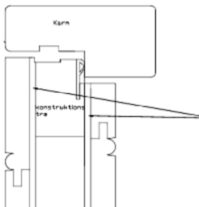
Fig. 2: Beklædning vist som både ind- og udadgående dør
