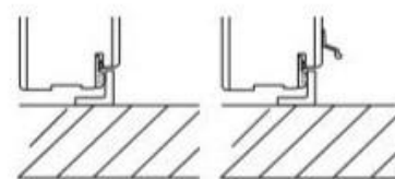
25x25 mm galv. vinkelskinne
