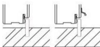
8x40 mm galv. bundskinne til nedstøbning
