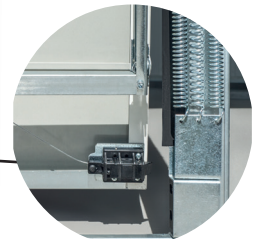
Låsefalle Lavet af forstærket plastik
